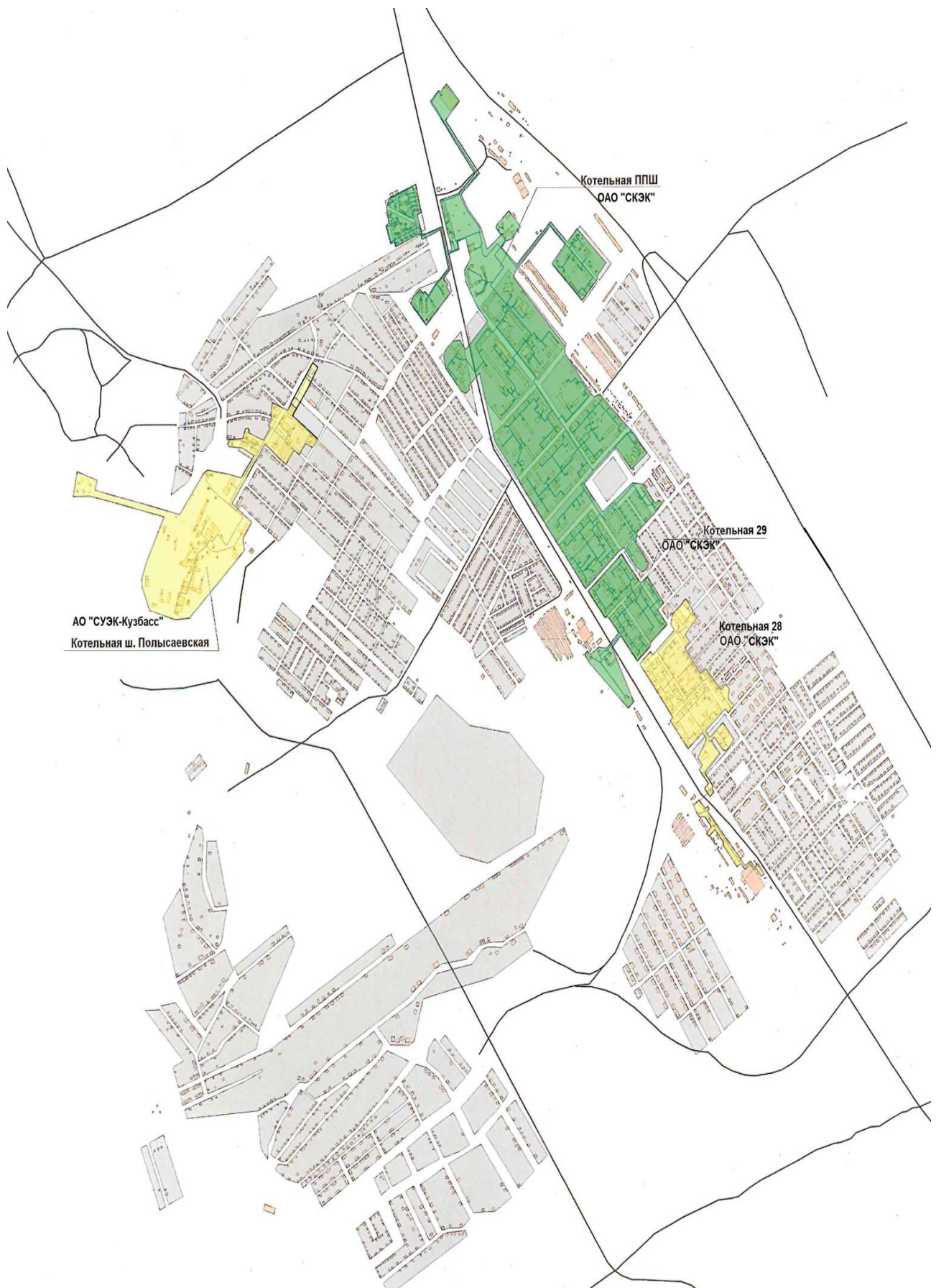
Рисунок 6. Схема тепловых сетей в зонах действия источников тепловой энергии Полысаевского городского округа
